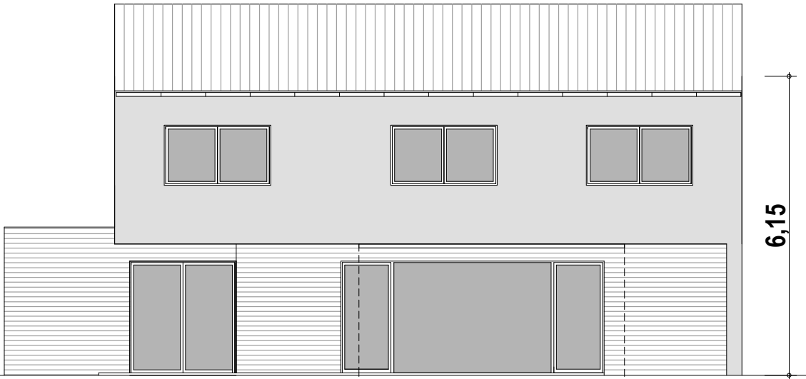
SÜDANSICHT
